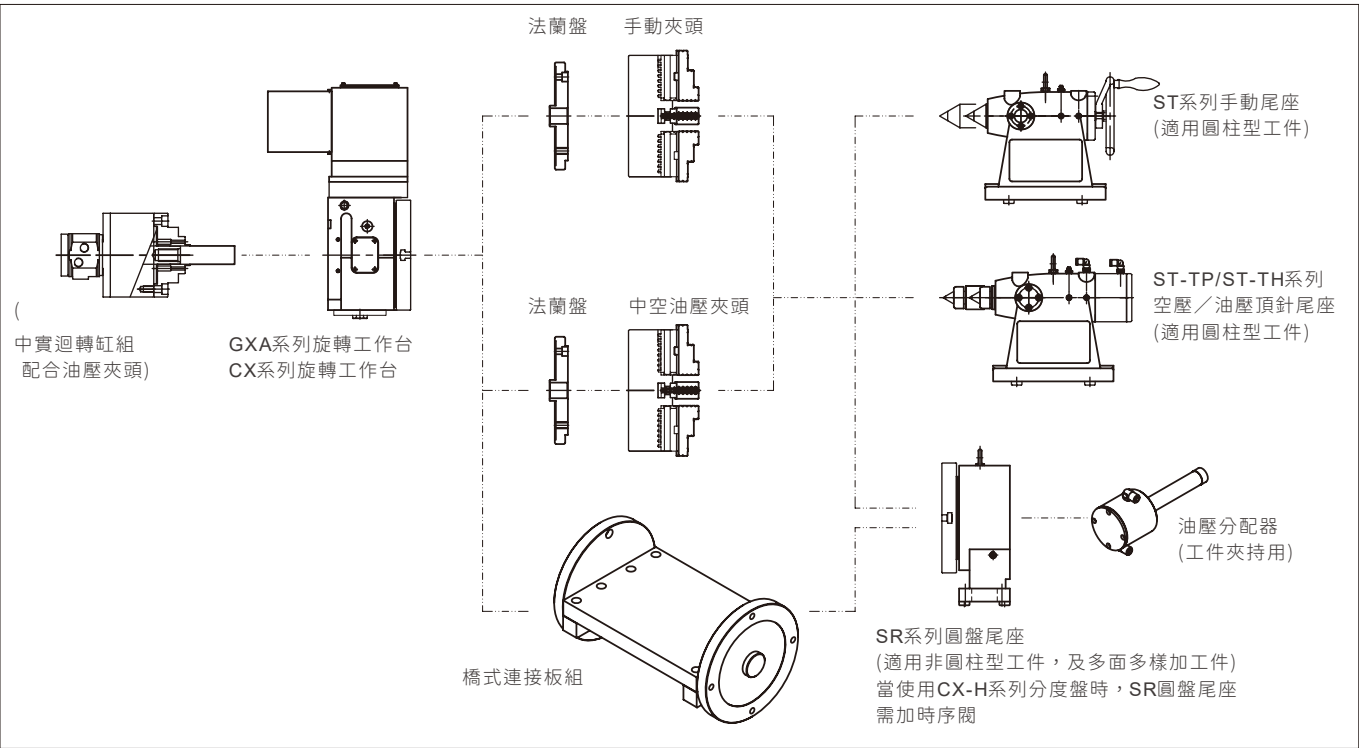
配件連接示意圖
